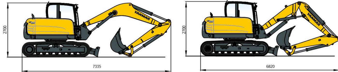
Abb. 2: Transportstellung
